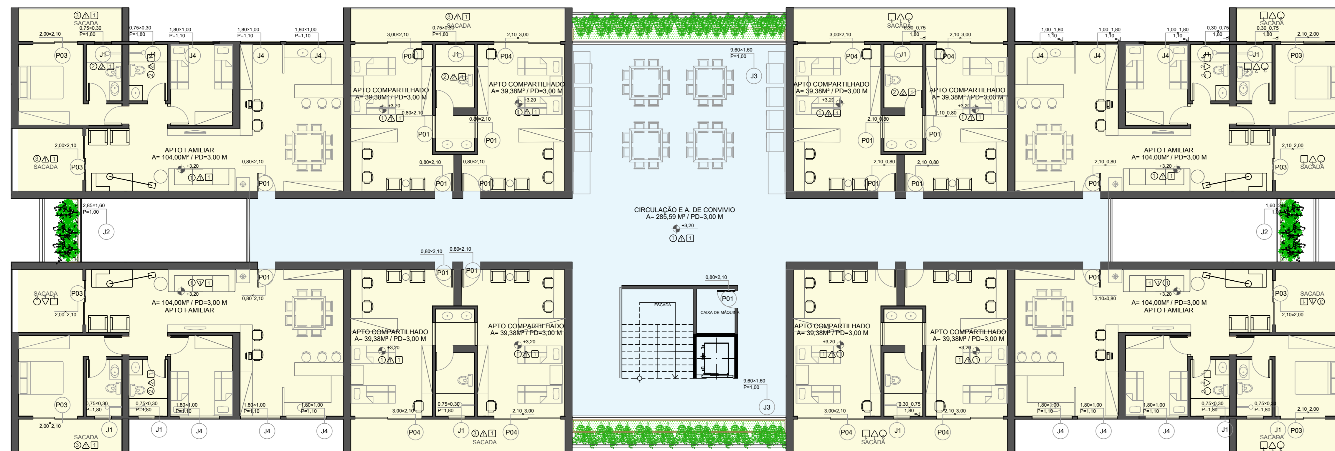
PLANTA PRIMEIRO PAVIMENTO TIPO (BLOCOS) Esc.: 1/100
