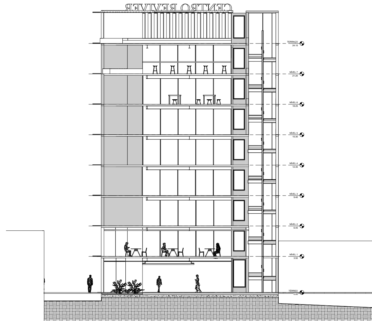
① CORTE AF 1:50
