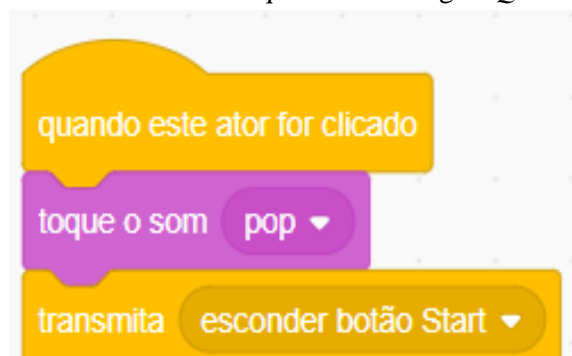
Figura 77 - Print Screen da interface da sequência de códigos ‘Quando este ator for clicado’
