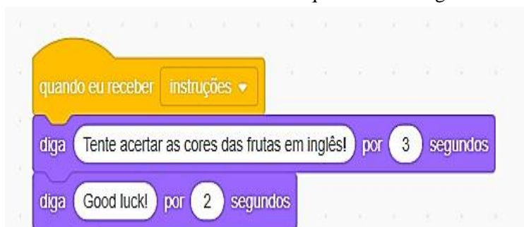
Figura 16 - Print Screen da interface da sequência de códigos das instruções
