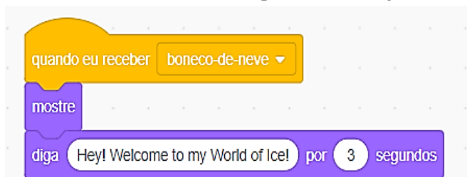
Figura 12 - Print Screen da interface da sequência de códigos do Boneco de Neve
