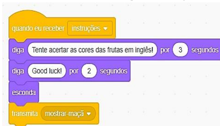
Figura 20 - Print Screen da interface da sequência de códigos das instruções
