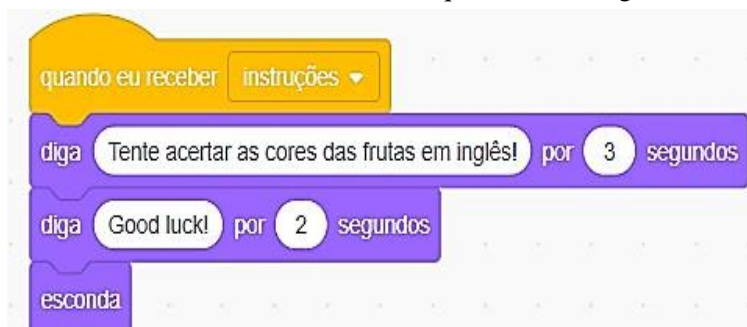
Figura 19 - Print Screen da interface da sequência de códigos das instruções
