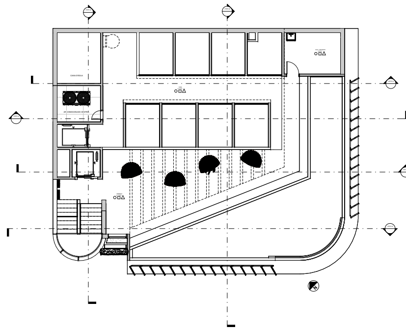
1 TERRAÇO 1:50
