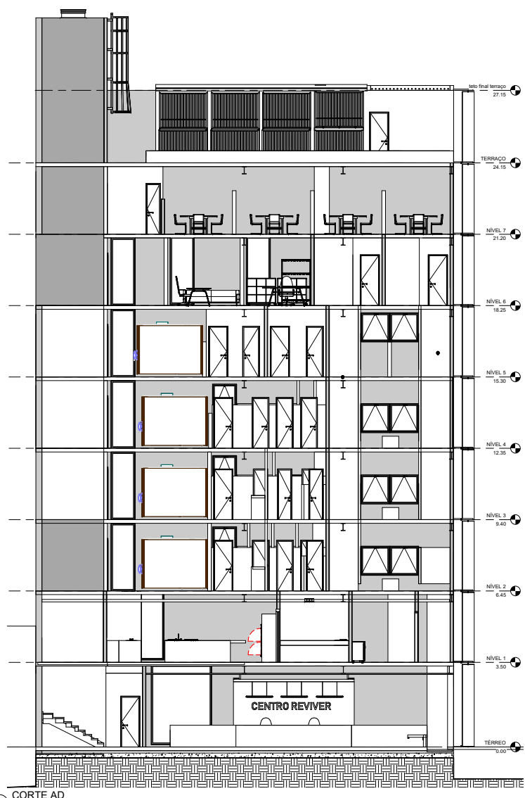
1 CORTE AD 1:50
