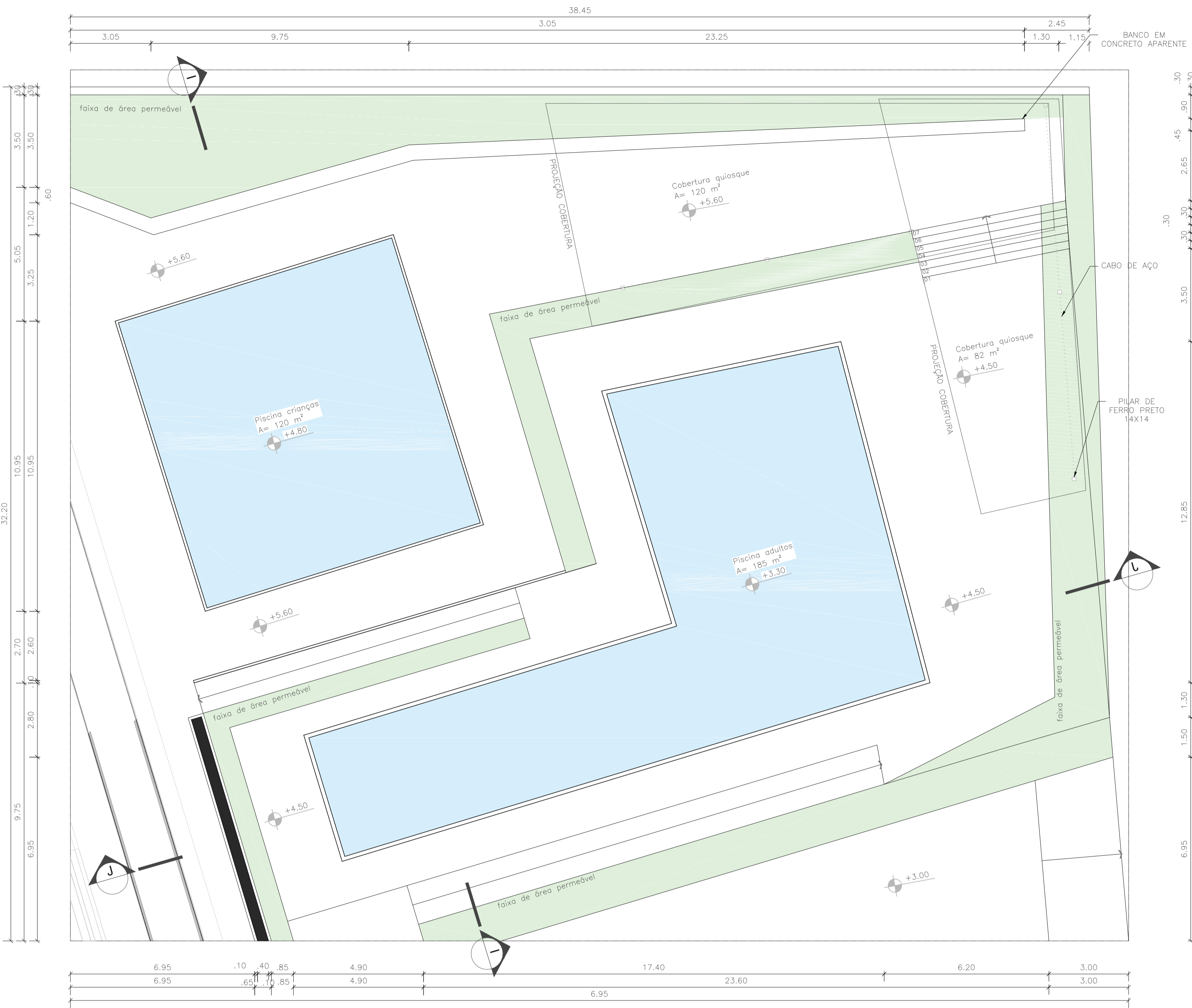
21 PISCINAS ABERTAS ESCALA 1:100
