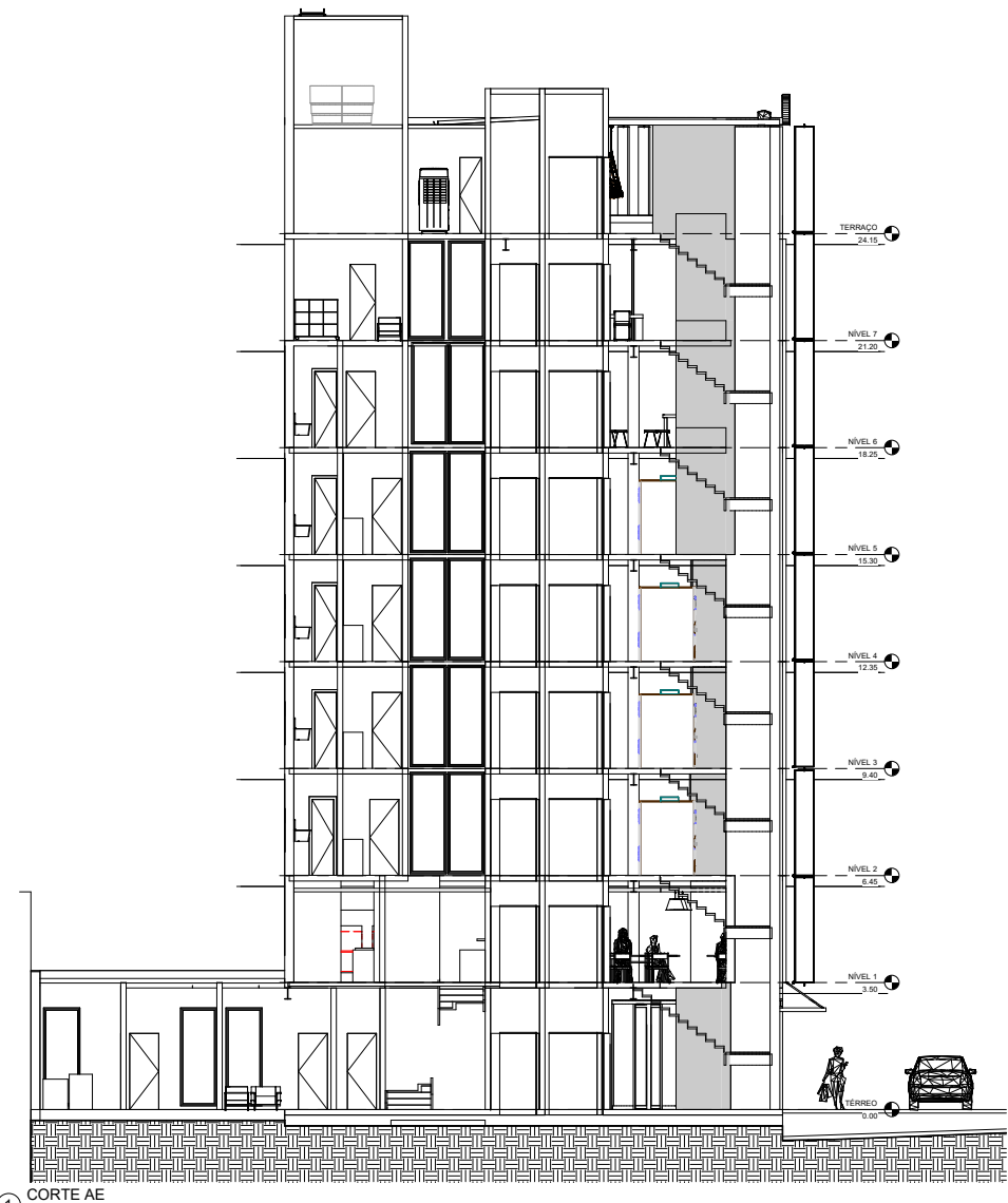
① CORTE AE 1:50
