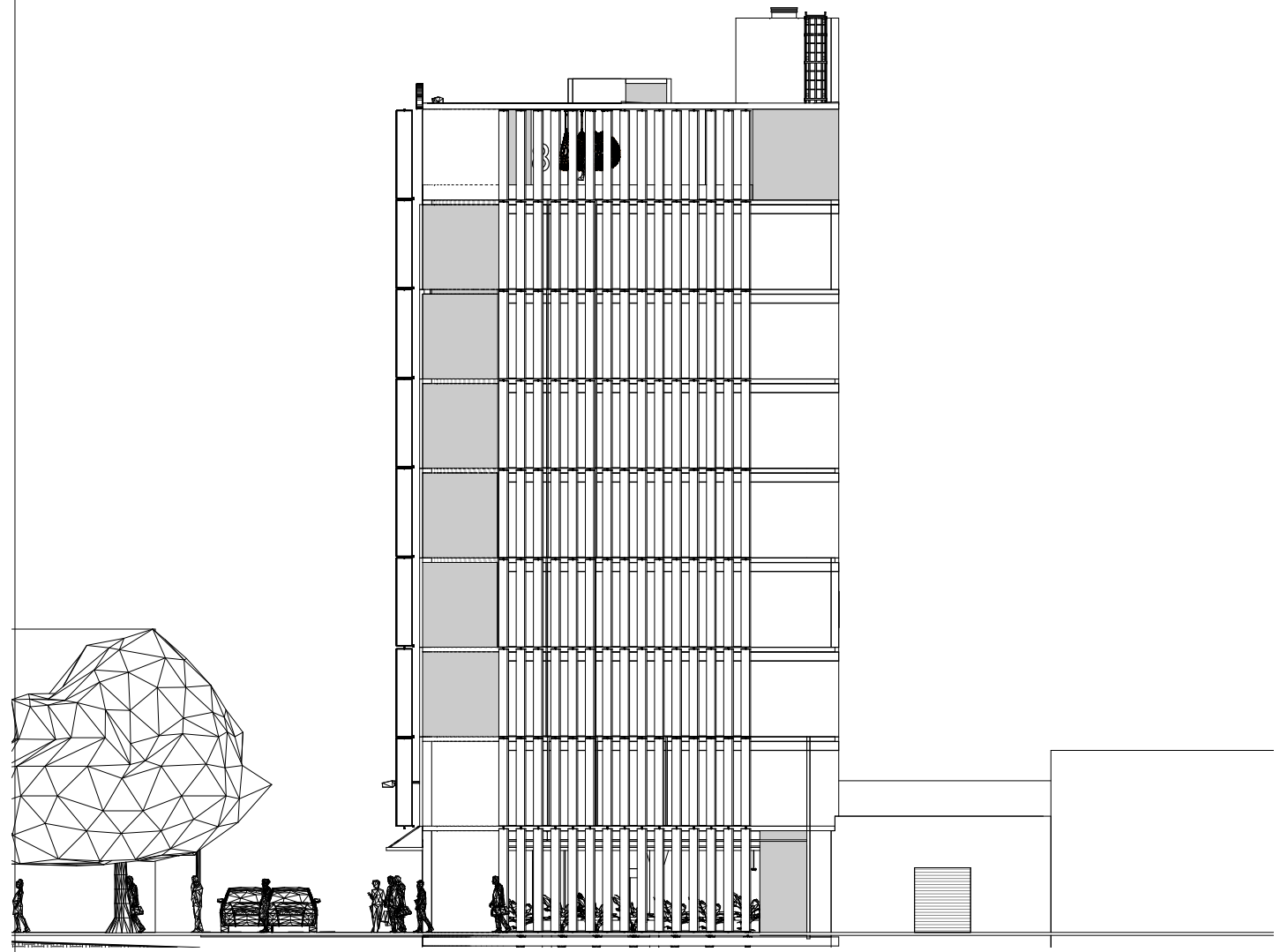
① ELEVACÃO OESTE 1:50
